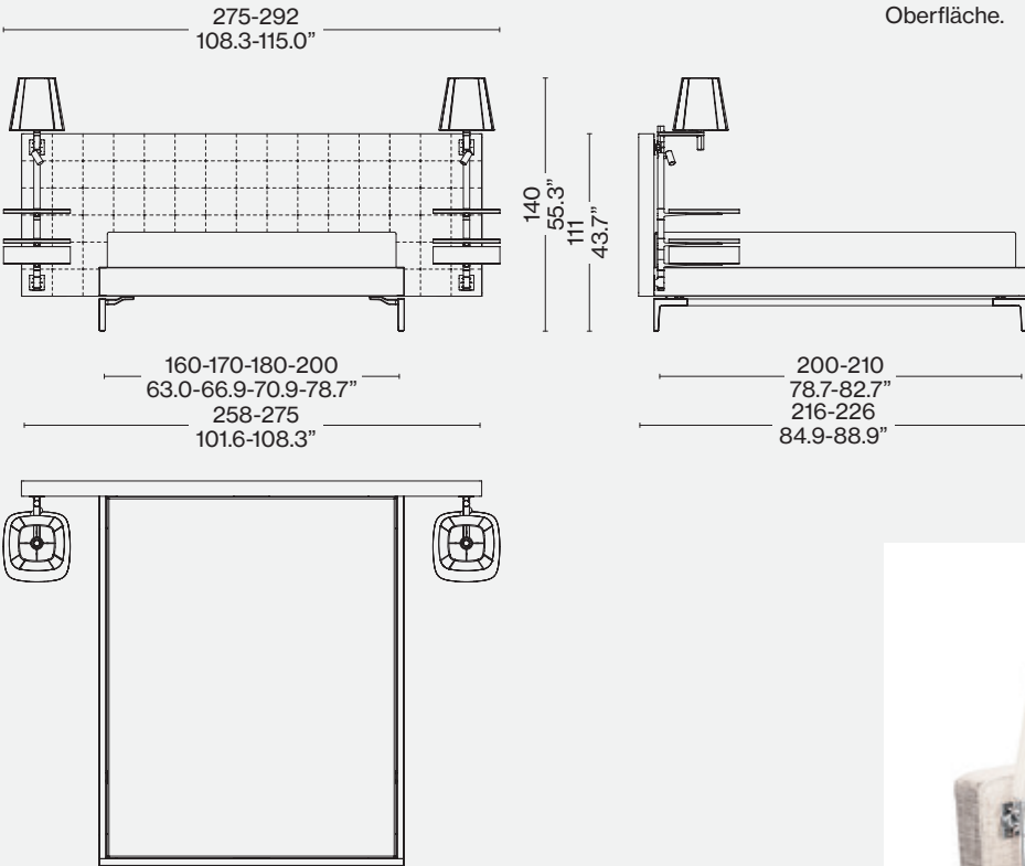
Misure giroletto - Rete/Sommier
