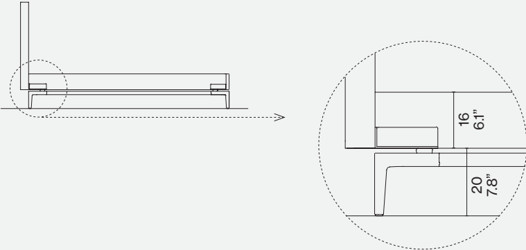
Misure giroletto - Rete/Sommier
